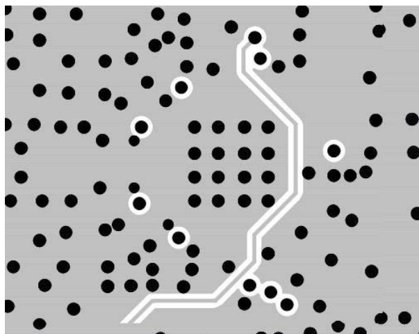
Inner Layer 3
